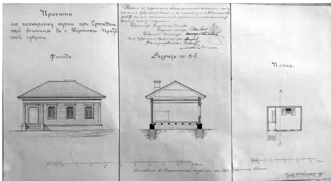
Рис. 5. Проект постройки кухни для Киренской гражданской больницы.
